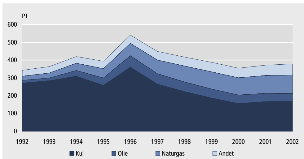
Figur 2. Kraftværkernes energiforbrug
