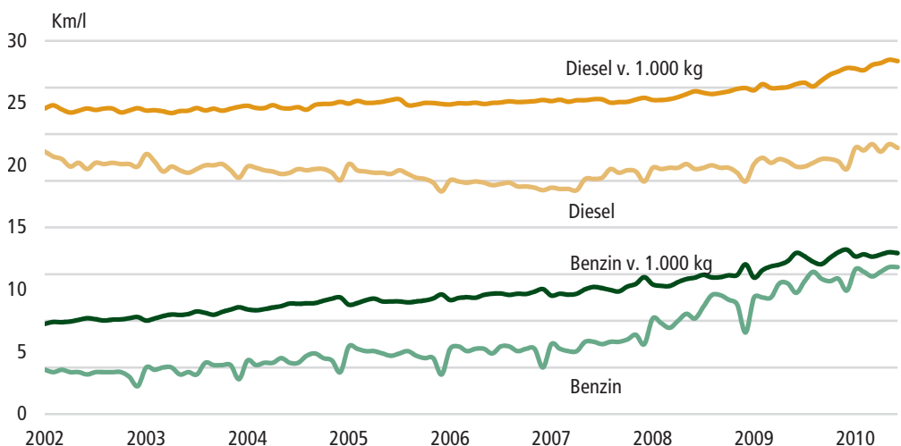
Figur 5 Energieffektiviteten for nyregistrerede personbiler
