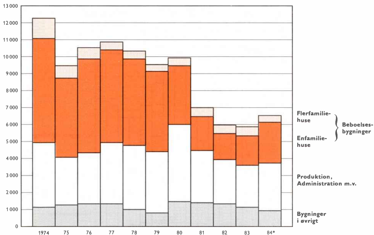
Fuldført byggeri (ekskl. sommerhuse) 1974-84*
