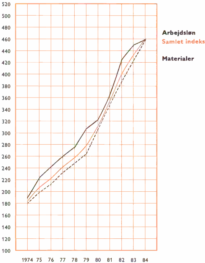
Byggeomkostningsindeks for et enfamiliehus (1/1-68=100) 1974-84
