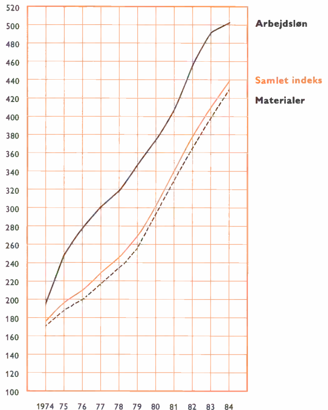
Byggeomkostningsindeks for en montagebygget ejendom (1/1-68=100) 1974-84
