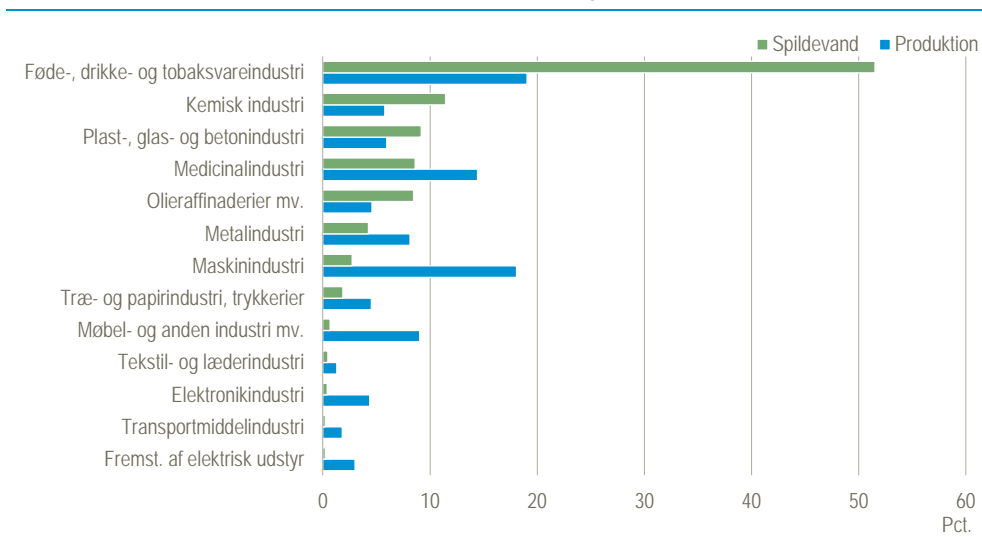
Figur 5.6 Industribrancherne andele af industriens spildevand og produktion. 2015
