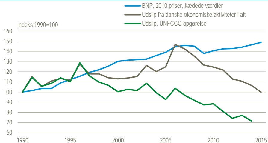
Figur 4.6. Udviklingen i bidrag til drivhuseffekten samt BNP
