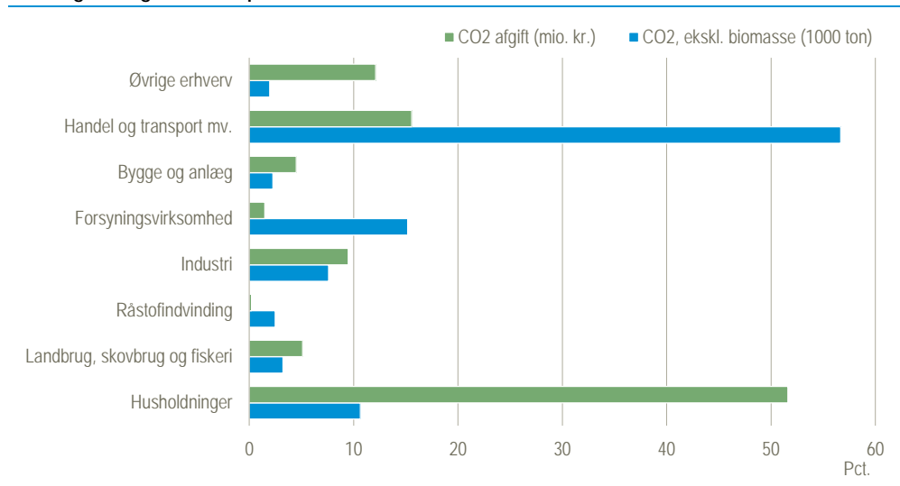
Figur 10.10 CO 2 -afgifter og CO 2 -udslip efter kilde. 2015
