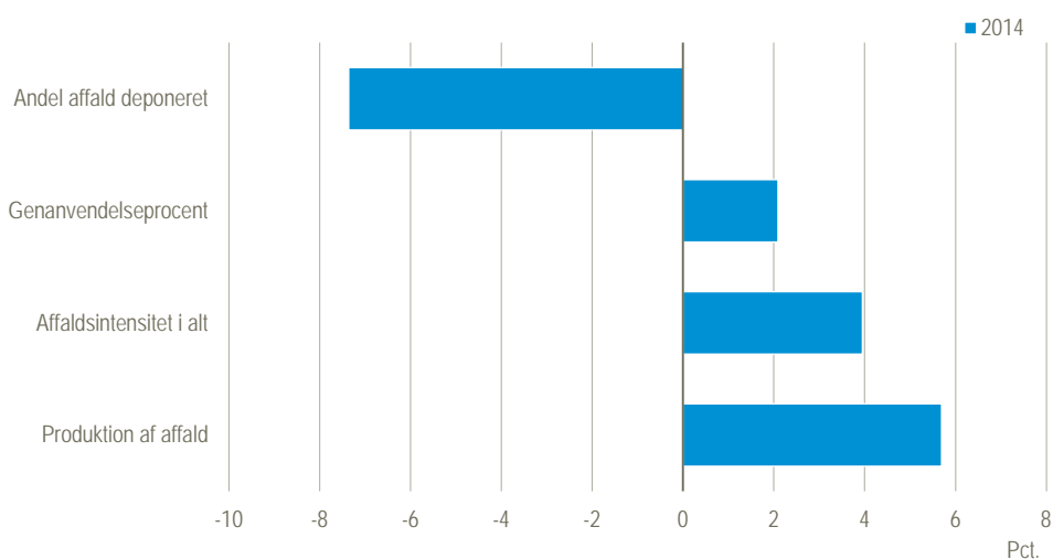
Figur 2.7 Udviklingen på affaldsområdet (procentvis ændring i forhold til året før)
