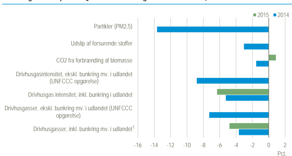
Figur 2.3 Udviklingen i udslip til luft (procentvis ændring i forhold til året før)
