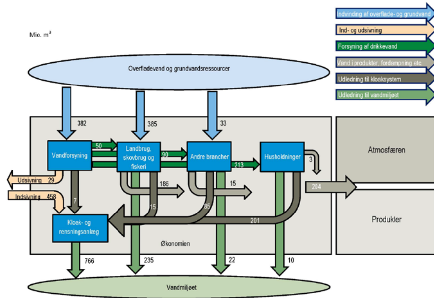
Figur 5.1 Strømme af vand og spildevand. 2015
