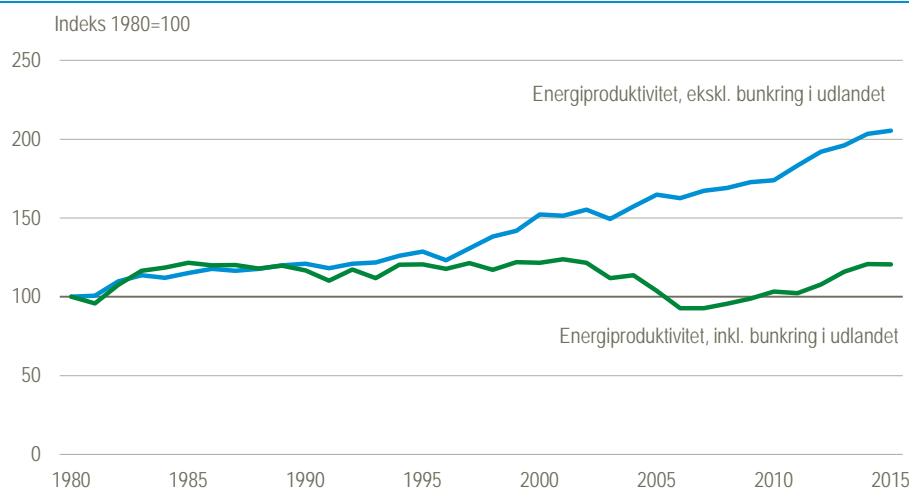
Figur 3.4 Indeks for energiproduktivitet, kr. BNP pr. GJ bruttoenergiforbrug
