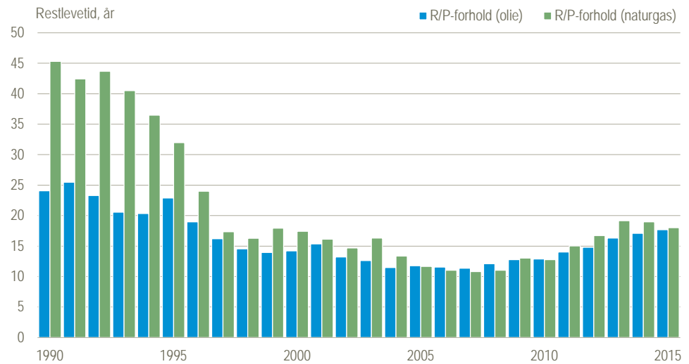
Figur 11.1 Reservernes restlevetid ved uændret produktion (R/P-forholdet)
