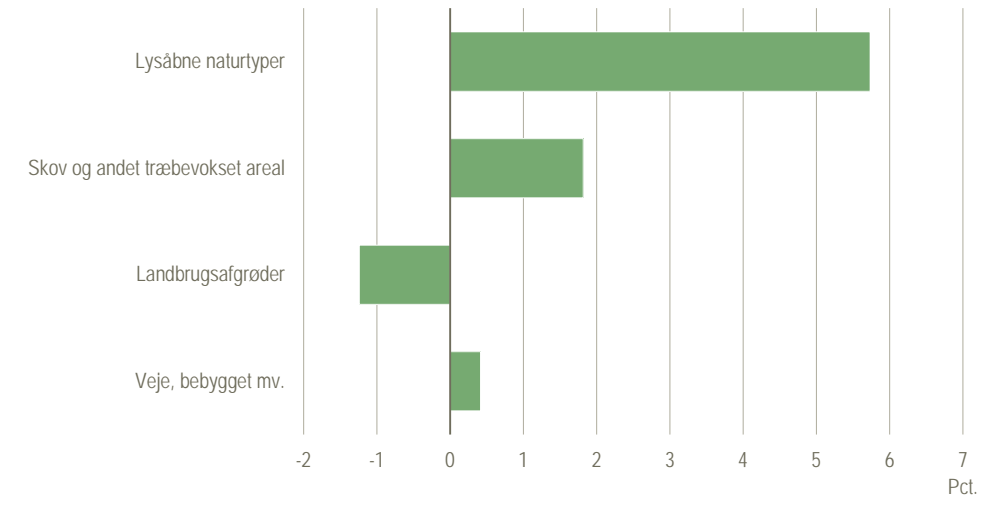
Figur 2.10 Udviklingen i vigtigste arealdækker (procentvis ændring 2011-2016)
