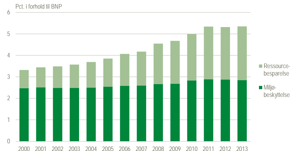
Figur 8.8 Omsætning af grønne varer og tjenester som andel af BNP, EU-28
