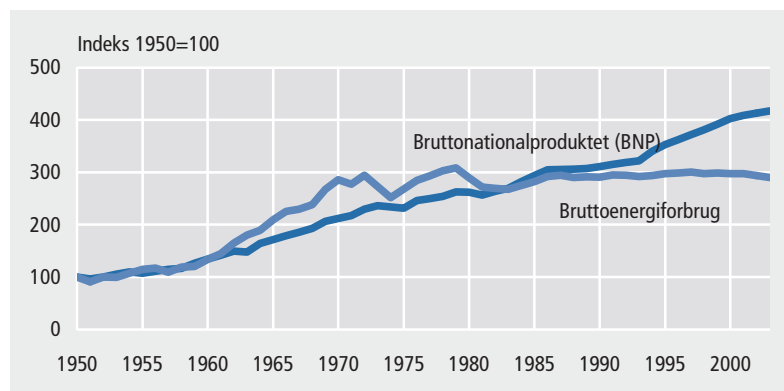
Figur 5.1 BNP i faste priser og bruttoenergiforbrug
