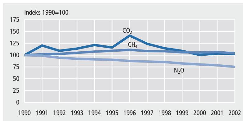
Figur 5.6 Samlet CO 2 -, CH 4 - og N 2 O-udslip
