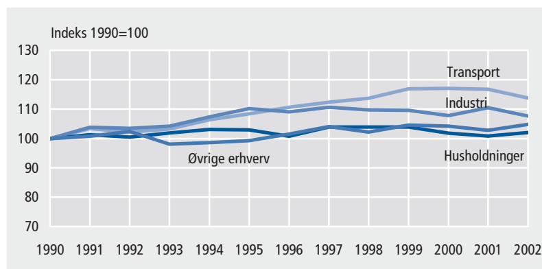
Figur 5.4 Endeligt energiforbrug fordelt på sektorer
