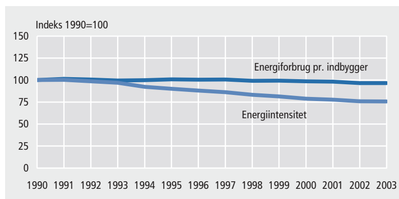
Figur 5.2 Energiintensiteten i Danmark og energiforbrug pr. indbygger
